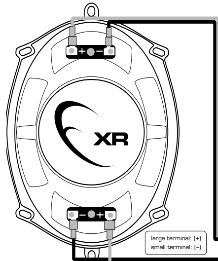
A) Wiring Diagram:
